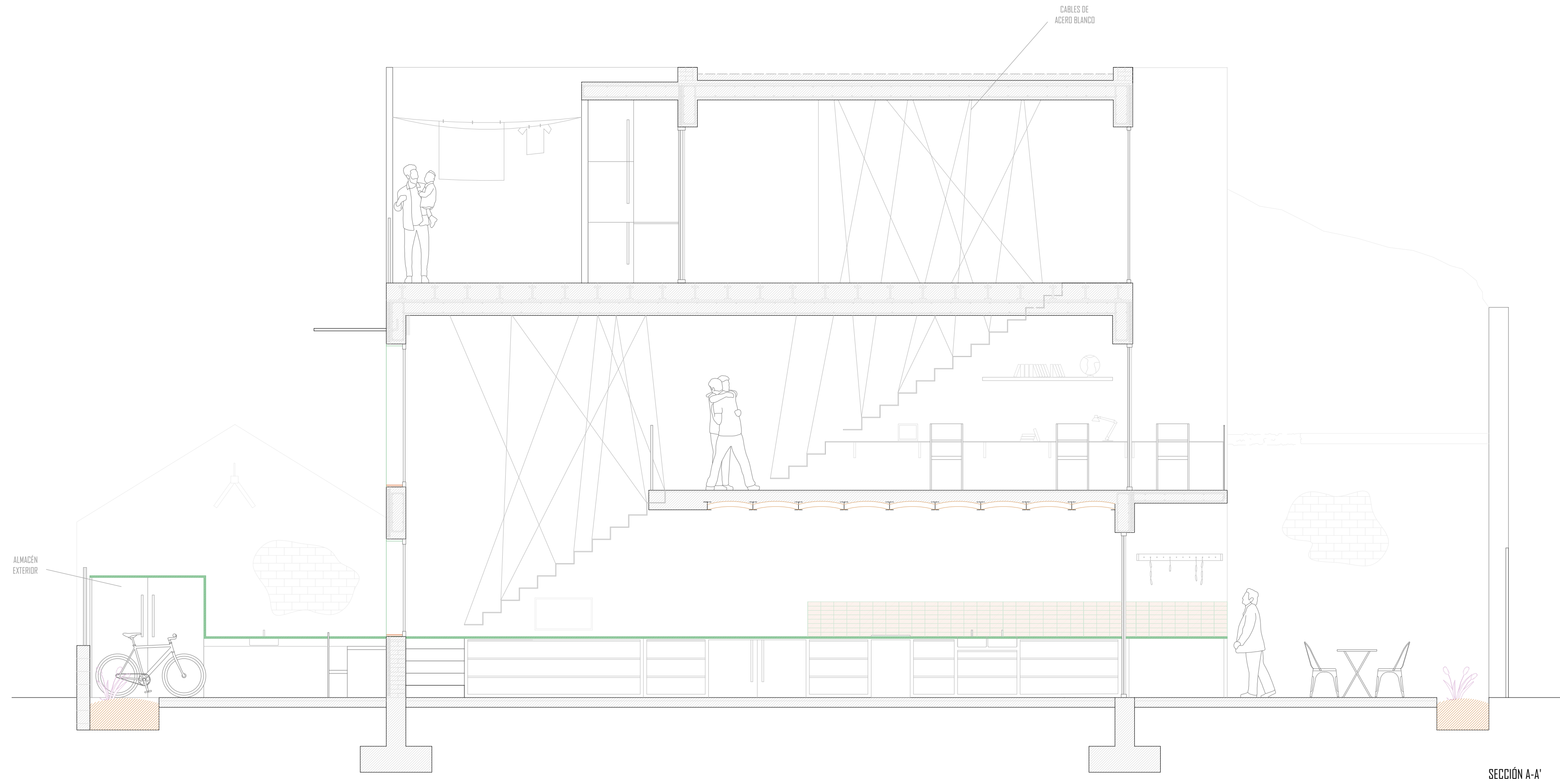
SECCIÓN A-A'
