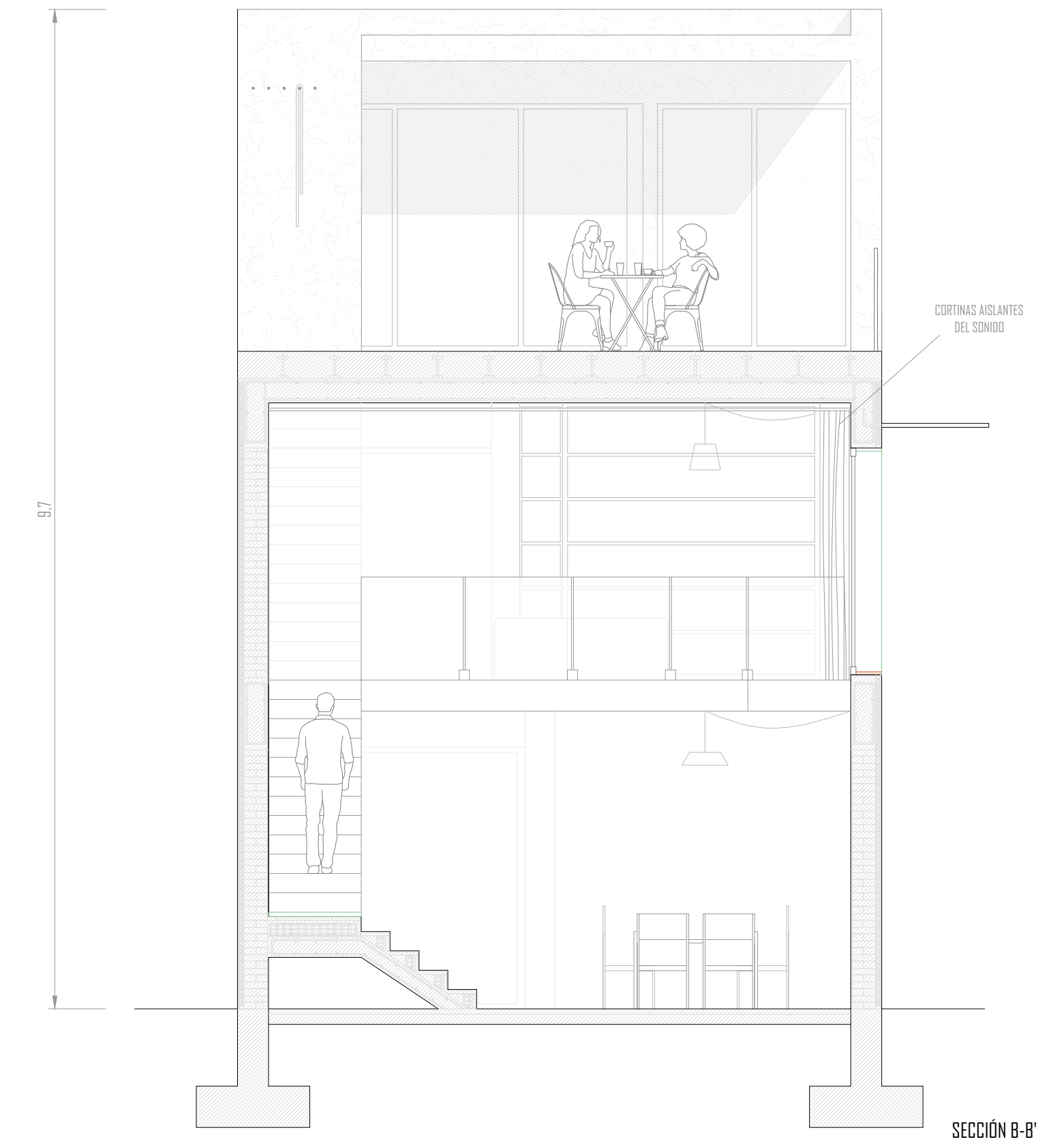
SECCIÓN B-B'
