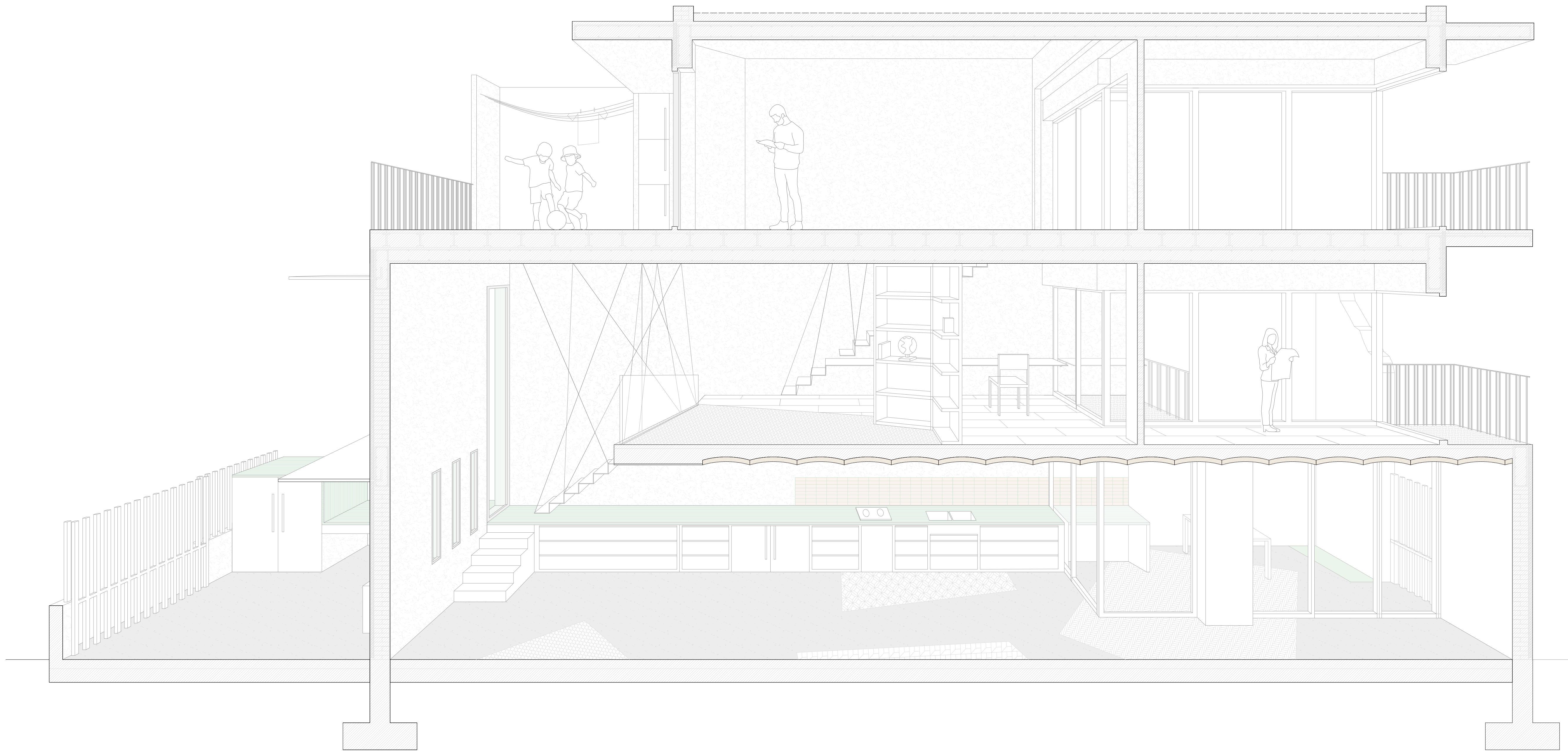
SECCIÓN 0-0'
