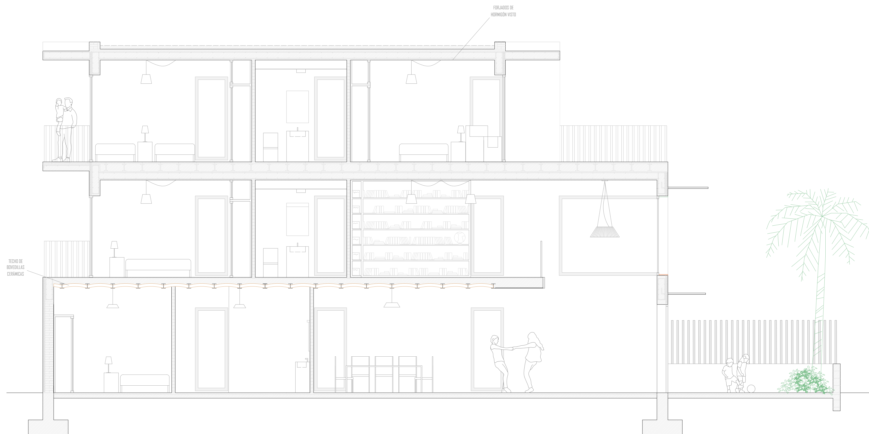
SECCIÓN C-C'
